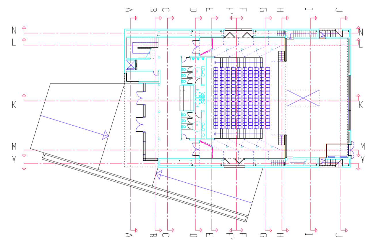
LLINEAS DE SECCIÓ EN PLANTA E= 1 / 250
