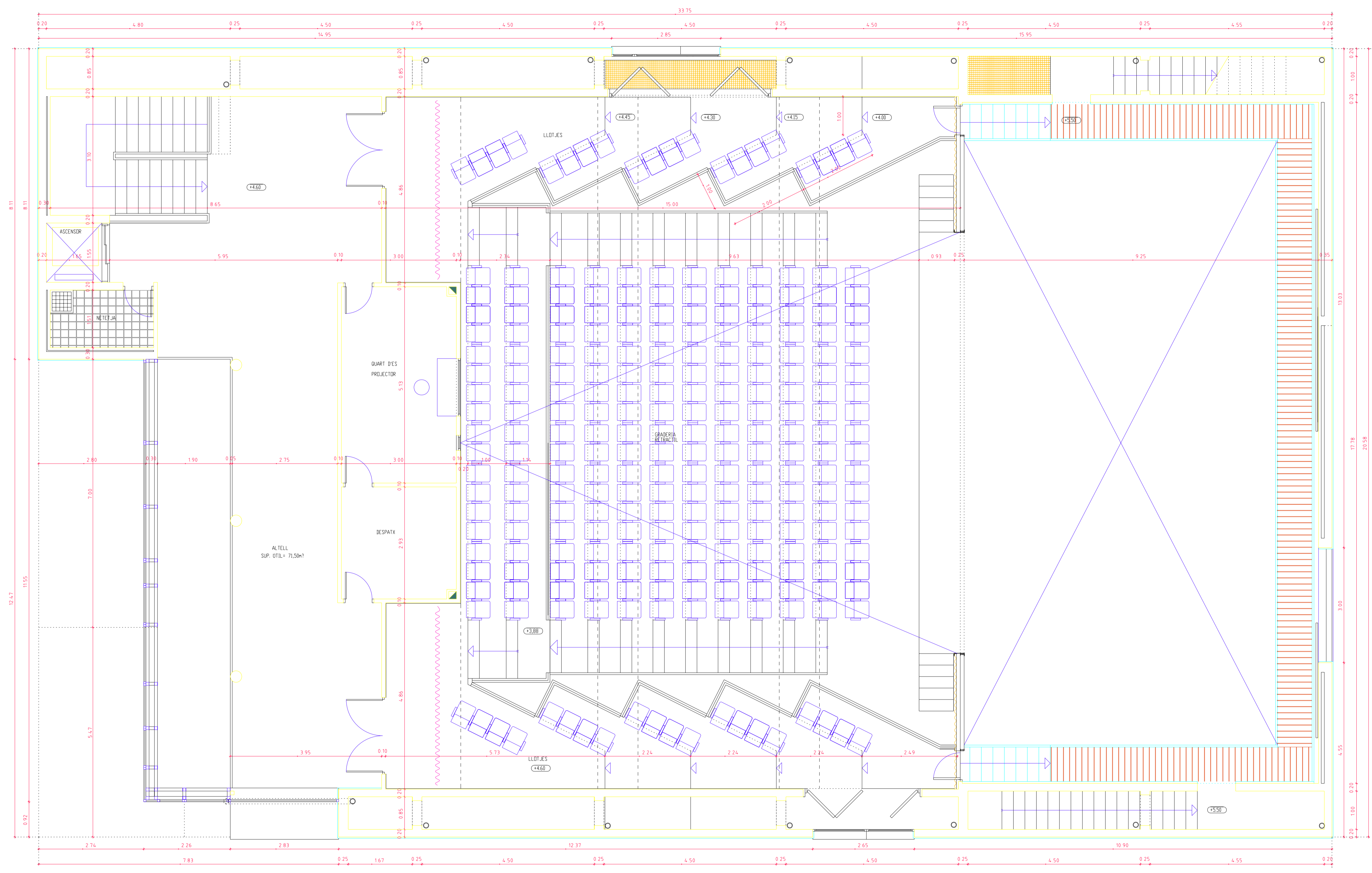
PLANTA ALTELL - LLOTJES E= 1/ 50
